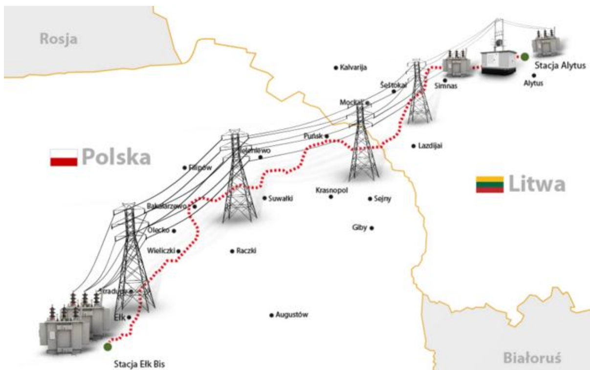
Rysunek 9. Przebieg linii Ełk – granica RP – Alytus ( www.litpol-link.com )
