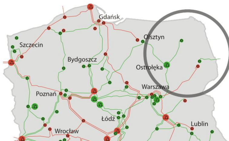
Rysunek 8. Mapa systemu przesyłowego w Polsce (kolor zielony – linia 220 kV, czerwony – linia 400 kV) ( www.liniaelgranica.pl )
